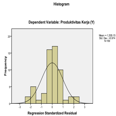
Gambar 4.2. Grafik Histogram
