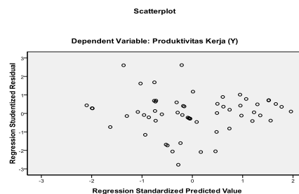
Gambar 4.4. Grafik Scatterplot
