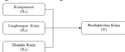
Gambar 2.1. Kerangka Konseptual
