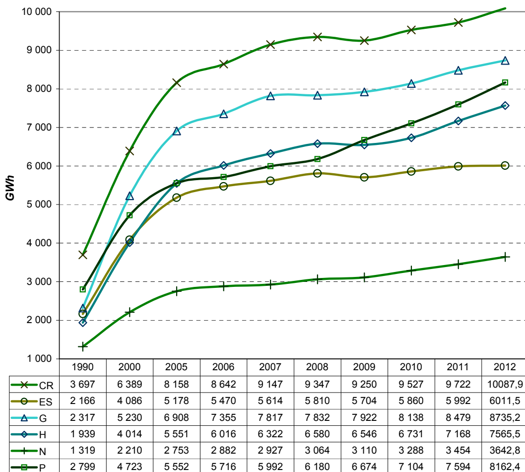
CUADRO 5 CENTROAMÉRICA: EVOLUCIÓN DE LA ENERGÍA ELÉCTRICA DISPONIBLE EN LOS MERCADOS NACIONALES, 1990-2012 a
