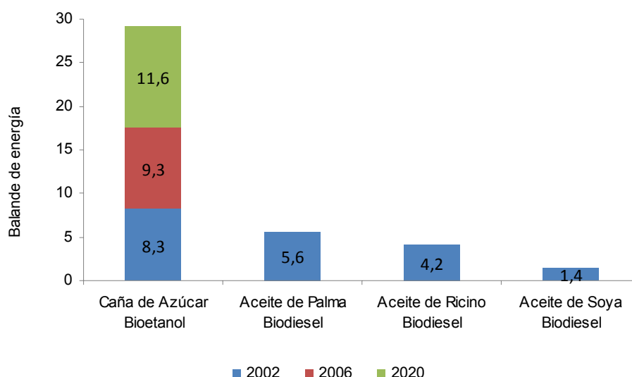
GRÁFICO V.1 BALANCE ENERGÉTICO BIOCMBUSTIBLES EN BRASIL
