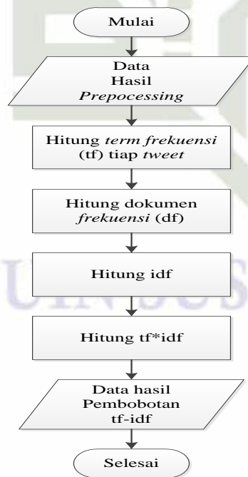
Gambar 3.3 Alur Pembobotan TF-IDF
