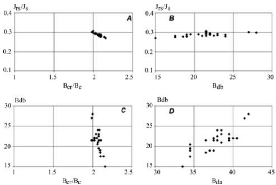
Рис. 4. Соотношение между гистерезисными параметрами образцов донных отложений оз. Большой Харбей (кern N): B_{db} – положение максимума производной dJ/dB_b (нормальное намагничивание вдоль оси b диаграммы Прейзаха-Нееля); остальные обозначения – см. рис. 3
