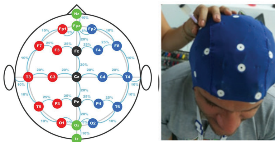
Figura 2. Protocolo 10/20 distancias del electrodo del sistema
