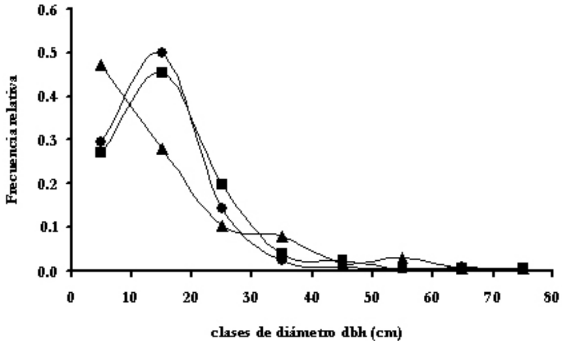
Figura 3. Frecuencia relativa de clases de diámetro (dbh) en las bandas altitudinales de 1000-1200m (puntos), 1200-1400 (cuadrados) y 1400-1600 (triángulos). En los tres casos la distribución observada se ajusta al modelo Log-normal (Test de Kolmogorov-Smirnov; \alpha < 0.05 ).
