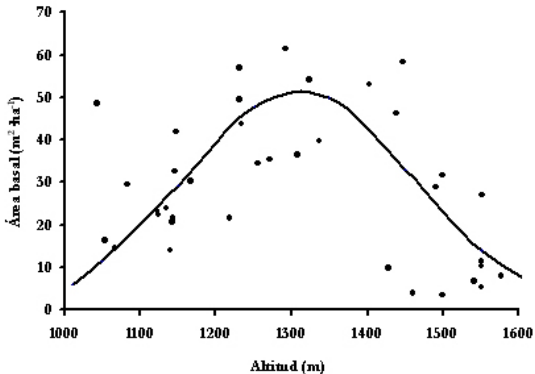
Figura 2. Densidad del pinsapar (m 2 ·ha -1 ) a lo largo del gradiente altitudinal; r=0.984.
