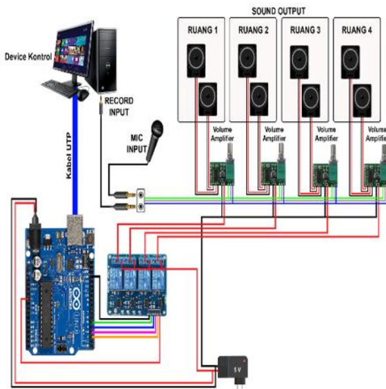
Gambar 14 Desain Sistem
