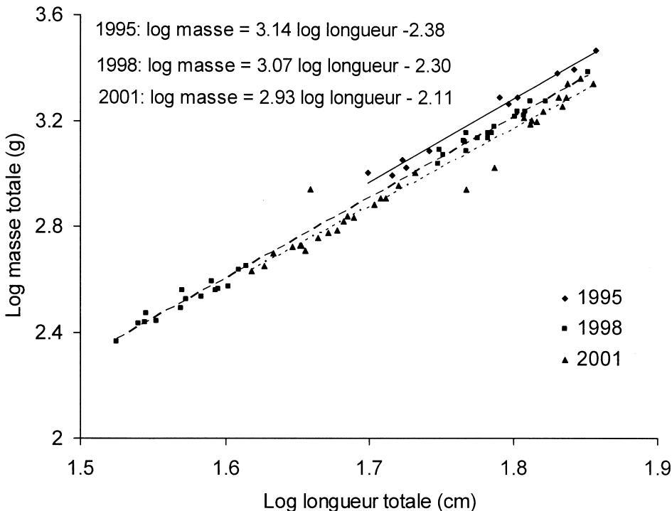
FIGURE 1. Relation logarithmique entre la masse totale et la longueur totale des Grands brochets du lac Ramsay. Le coefficient de condition correspond à la pente des droites. 1995 : n = 11 ; 1998 : n = 34 ; 2001 : n = 32.
