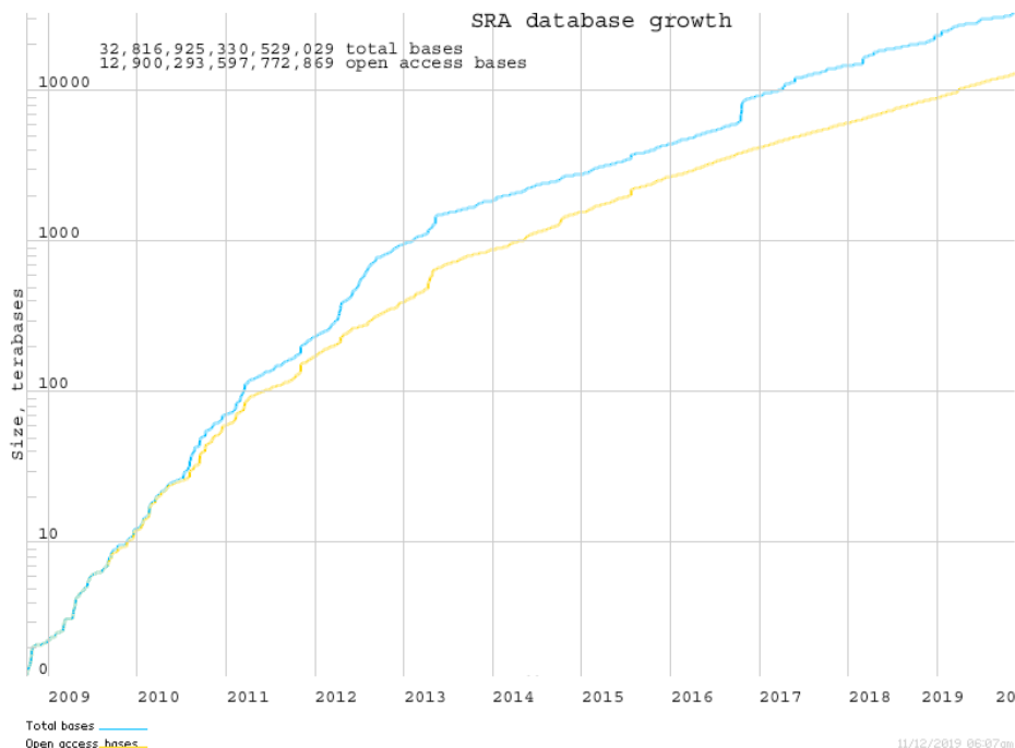
図 1: SRA に登録されたデータ量の変化
