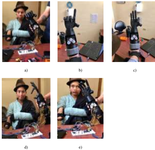
Figura 51-3. Pruebas en el prototipo: a) Dedos cerrados – Gesto Puño. b) Dedo índice abierto. c) Cerrar dedo pulgar e índice. d) Giro de la muñeca 90° – Gesto Mano hacia adentro. e) Dedos Abiertos y muñeca en posición inicial.
