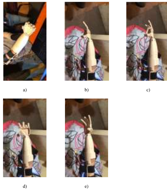
Figura 52-3. Pruebas en la prótesis: a) Dedos cerrados – Gesto Puño. b) Dedo índice abierto. c) Cerrar dedo pulgar e índice. d) Giro de la muñeca 90° – Gesto Mano hacia adentro. e) Dedos Abiertos y muñeca en posición inicial.
