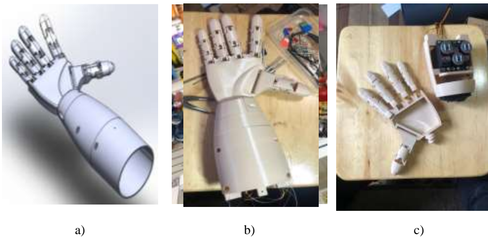
Figura 38-3. a) Diseño de la prótesis. b) Prótesis impresa. c) Colocación de los servomotores
