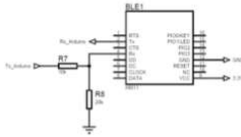
Figura 30-3. Esquema de conexión HM-11 y Placa Arduino
