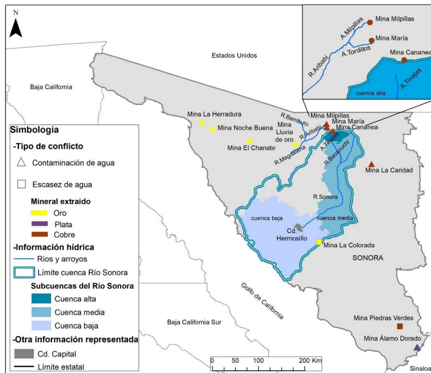
FIGURA 2 – Conflictos por agua en minas de tajo a cielo abierto.
