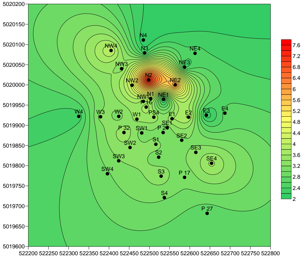
Figura 18. Distribuzione del C (%) totale nel sito PS 4
