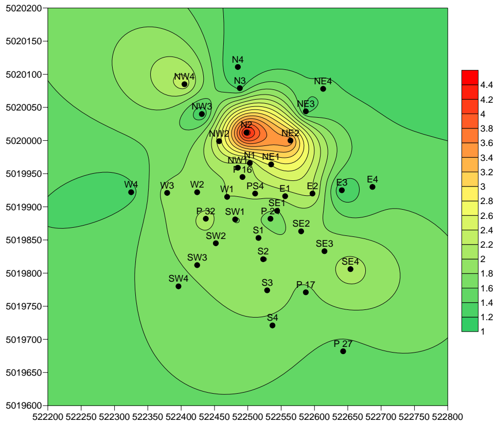
Figura 19. Distribuzione del C organico (%) nel sito PS 4
