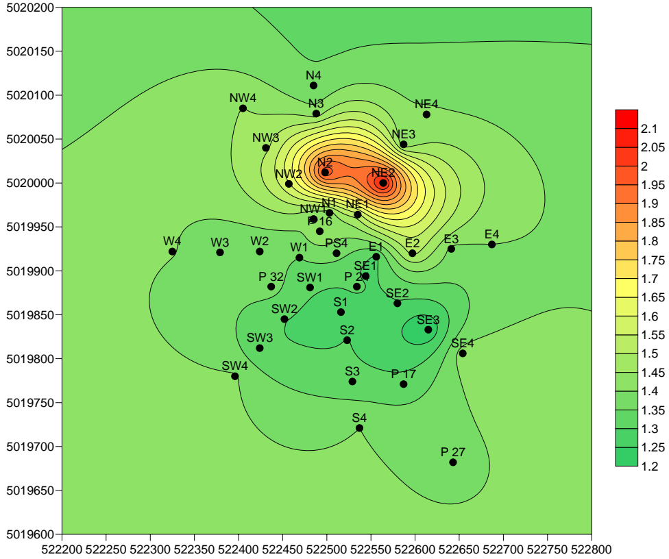
Figura 17. Distribuzione di Ca (%) nel sito PS 4
