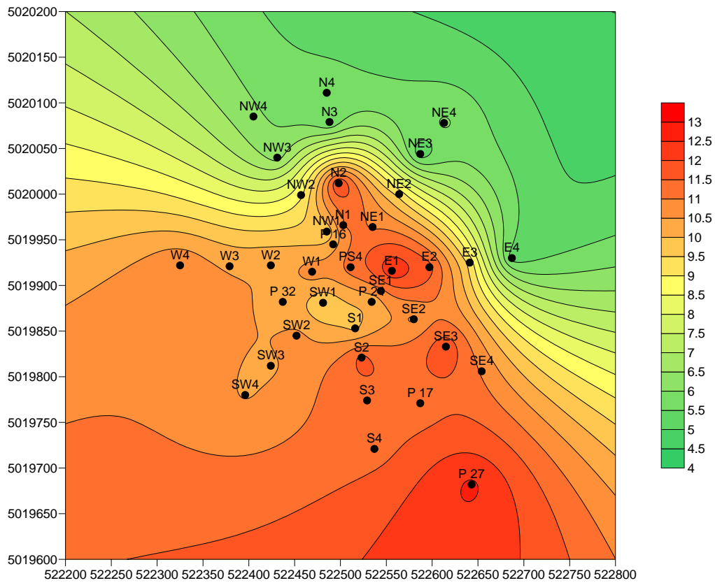
Figura 23. Distribuzione di Co ( \mu\text{g/g} ) nel sito PS 4
