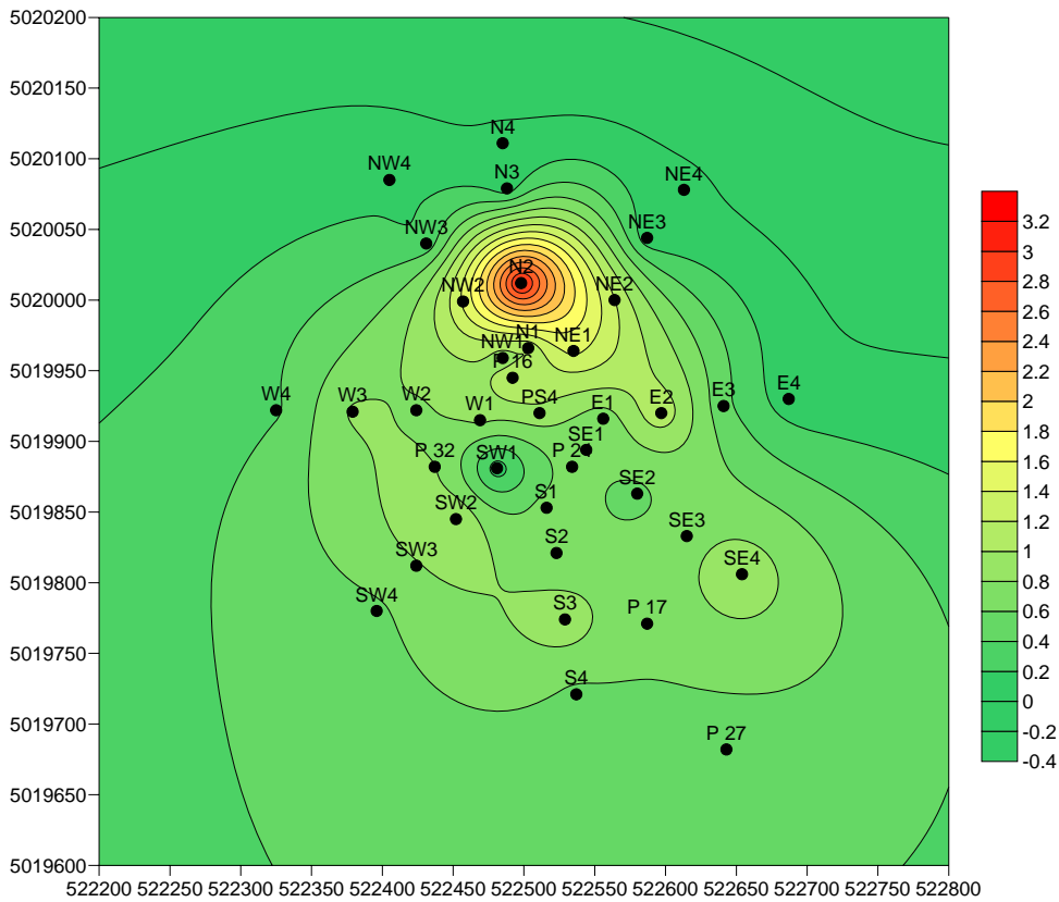
Figura 11. Distribuzione di Hg (µg/g) nel sito PS 4
