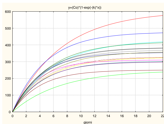
Figura 6. Curve cinetiche dell'attività di mineralizzazione potenziale della sostanza organica disegnate secondo il modello cinetico esponenziale y=Ct = C0(1-\exp(-kt)) . Le curve colorate in figura corrispondono ai seguenti campioni: N4-SE4-P24-P17-NE4-NE1-E2-P32-P27-P16-N1-W1-PS4-NW2-NE2-N2
