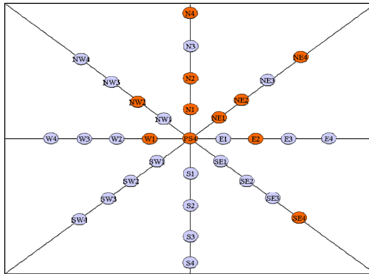
Figura 1 – disposizione dei punti di campionamento attorno al punto 4PS. I campioni segnati in arancio sono stati analizzati anche dal punto di vista biochimico.
