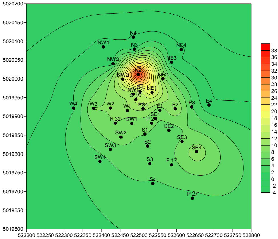
Figura 10. Distribuzione di Cd (µg/g) nel sito PS 4
