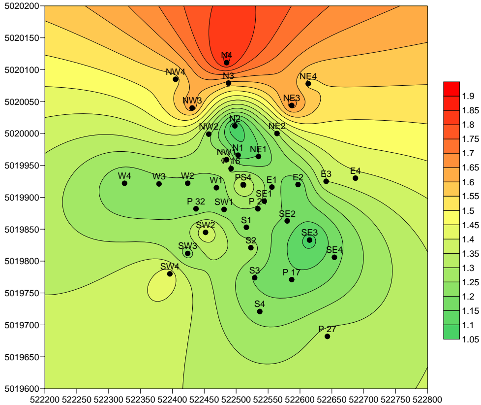
Figura 31. Distribuzione di Na (%) nel sito PS 4
