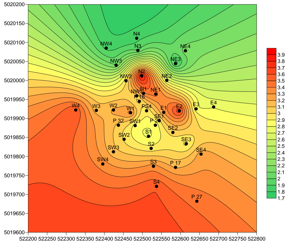
Figura 21. Distribuzione di Fe (%) nel sito PS 4
