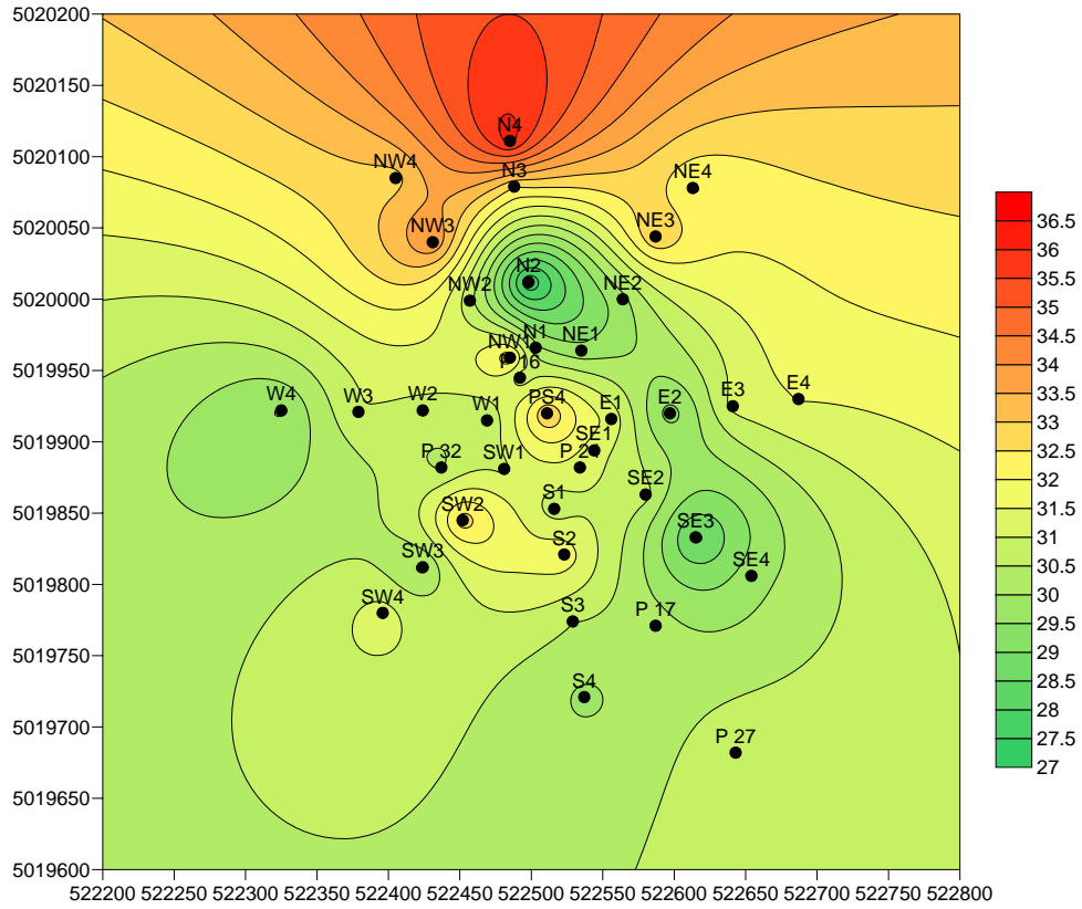
Figura 30. Distribuzione di Si (%) nel sito PS 4
