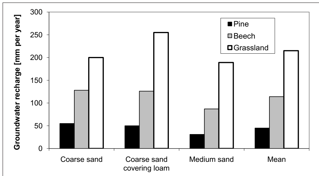
Fig. 3 Simulated annual mean groundwater recharge for different land-use scenarios and soils in the Schorfheide region 1952-2007 (source: Natkhin 2011) / Simulierte jährliche Grundwasserneubildung für verschiedene Landnutzungsszenarien und Böden in der Schorfheide 1952-2007 (Quelle: Natkhin 2011)
