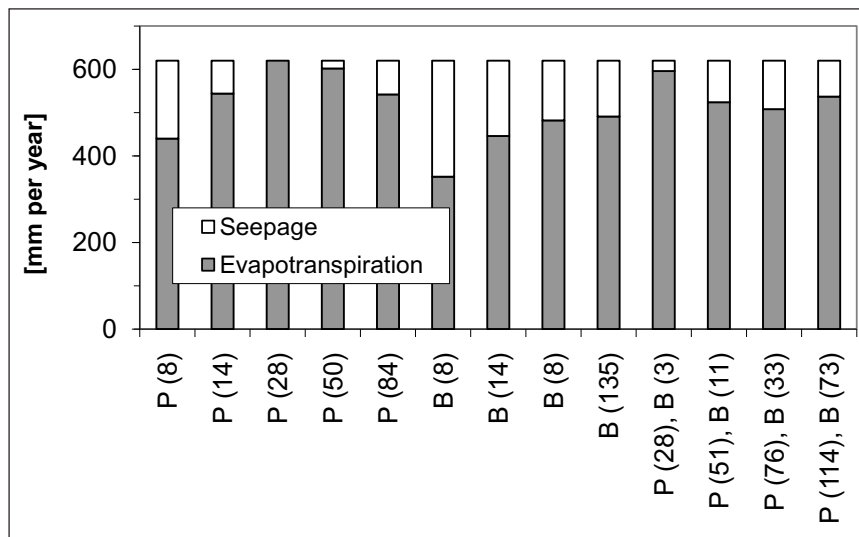
Fig. 4 Water budgets of different forests at a site close to Eberswalde with 620 mm per year mean annual precipitation. "P" denotes pine, "B" beech. In addition, tree age [years] is given in brackets. Data provided by Müller 2002 / Wasserbilanz für verschiedene Forstbestände nahe Eberswalde mit 620 mm/a Jahresniederschlag . „P“ steht für Kiefer, „B“ für Buche. Außerdem ist das Baumalter [Jahre] in Klammern angegeben. Datengrundlage: Müller 2002
