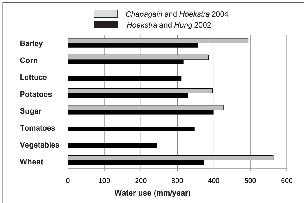
Fig. 5 Assessment of annual water use by different crops in Germany in two studies / Abschätzung des jährlichen Wasserverbrauchs durch unterschiedliche Feldfrüchte in Deutschland in zwei verschiedenen Studien
