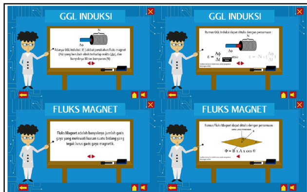
Gambar 14. Halaman Materi
