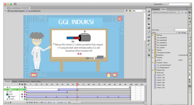
Gambar 10. Proses Animasi
