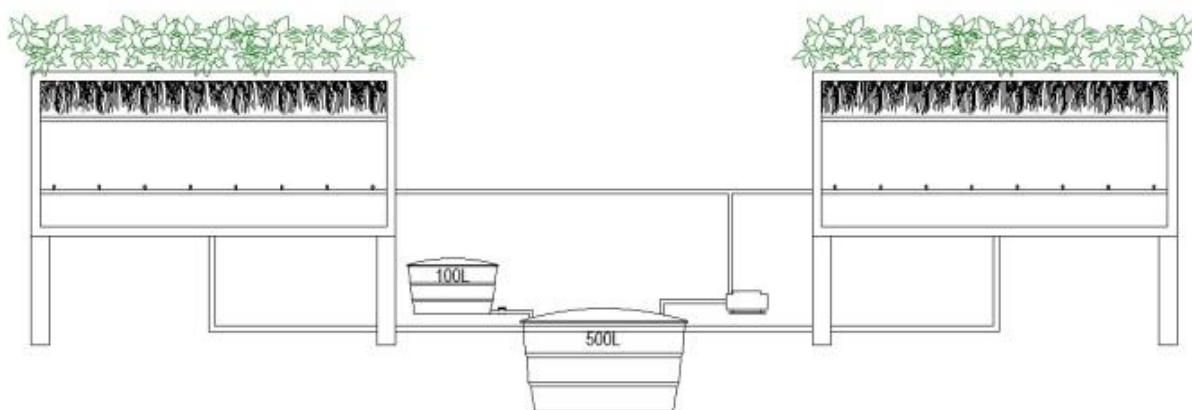
Figura 1. Esquema representativo das estruturas aeropônicas utilizadas no desenvolvimento do experimento de produção de batata-semente. Fonte: Tartaro et al. (2020).
