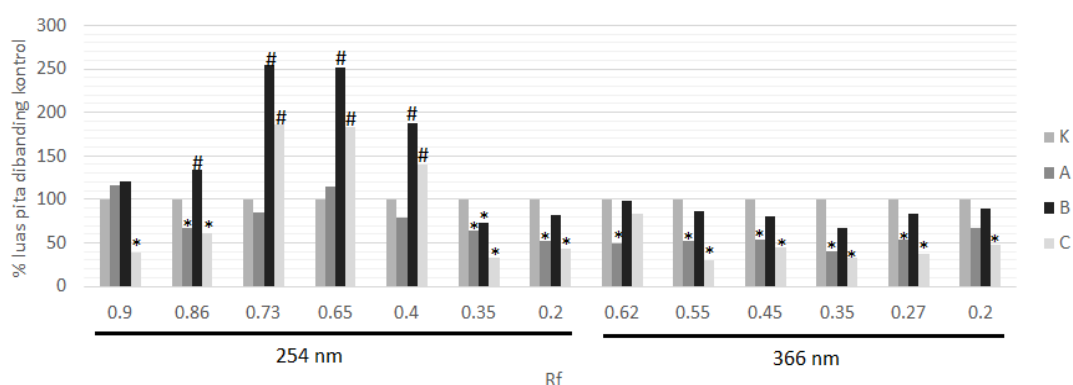
Gambar 5. Persentase perubahan luas pita pada Rf tertentu pada daun teh kontrol (K), teh dengan benalu A (A), teh dengan benalu B (B), dan teh dengan benalu C (C) dengan deteksi 254 nm dan 366 nm; Ket: #signifikan meningkat dibandingkan kontrol dan *signifikan menurun dibandingkan kontrol
