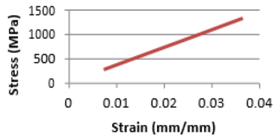
Gambar 5. Kurva Stress—Strain pada variasi [0/+45/+45/0]2s (atas) dan [0/+45/+90/-45]2s (bawah).
