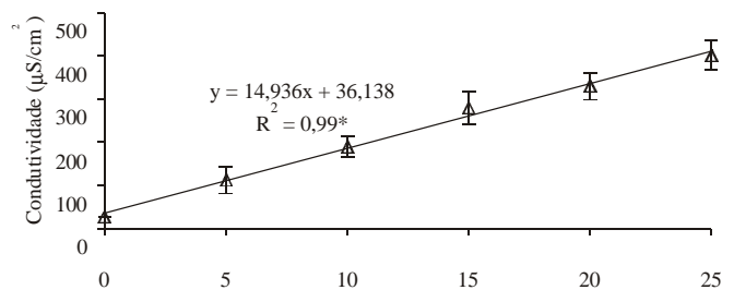
Figura 1. Variação (média±desvio-padrão) da condutividade da água em razão da concentração de amônia total em tanques experimentais de exposição de juvenis de pirarucu ( Arapaima gigas ) a um gradiente positivo de concentração de amônia na água (pH, 6,6 \pm 0,2 e temperatura, 26,9 \pm 0,9^\circ\text{C} ). *Significativo a 5% de probabilidade.
