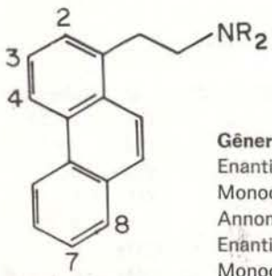
Tipo fenantrênico
