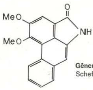
Tipo lactama
