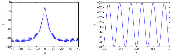
Figura 1 – À esquerda temos uma função unimodal, com um valor de ótimo bem destacado; Já à direita, temos uma função simétrica e multimodal (6 soluções ótimas).
