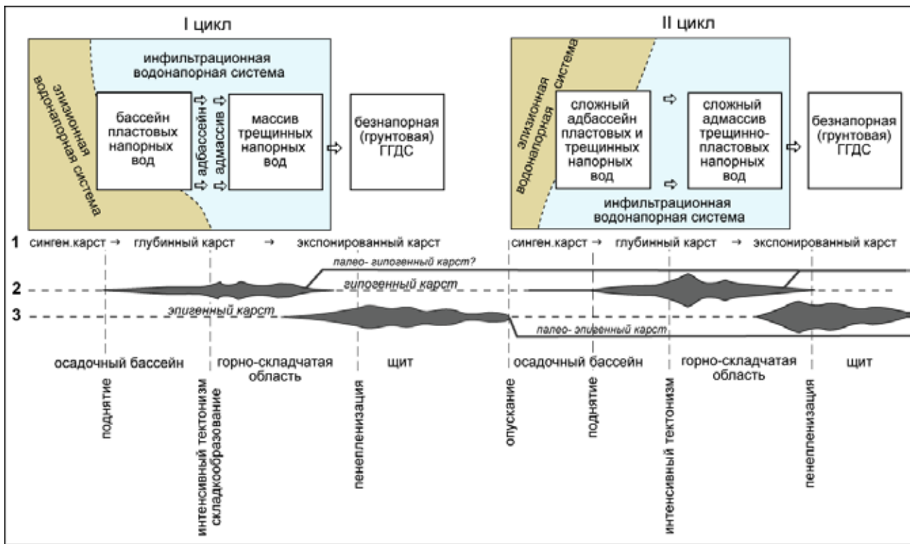
Рис. 1. Развитие карста в контексте эволюции геогидродинамических систем и гидрогеологических структур. Содержательная основа рисунка в общегидрогеологической части – по Карцеву (1972), с изменениями. Цифрами обозначены: 1 = направленность смены эволюционных типов (групп типов) карста; 2-3 = относительная интенсивность развития карста в ходе эволюции: 2 = гипогенного, 3 = эпигенного.
