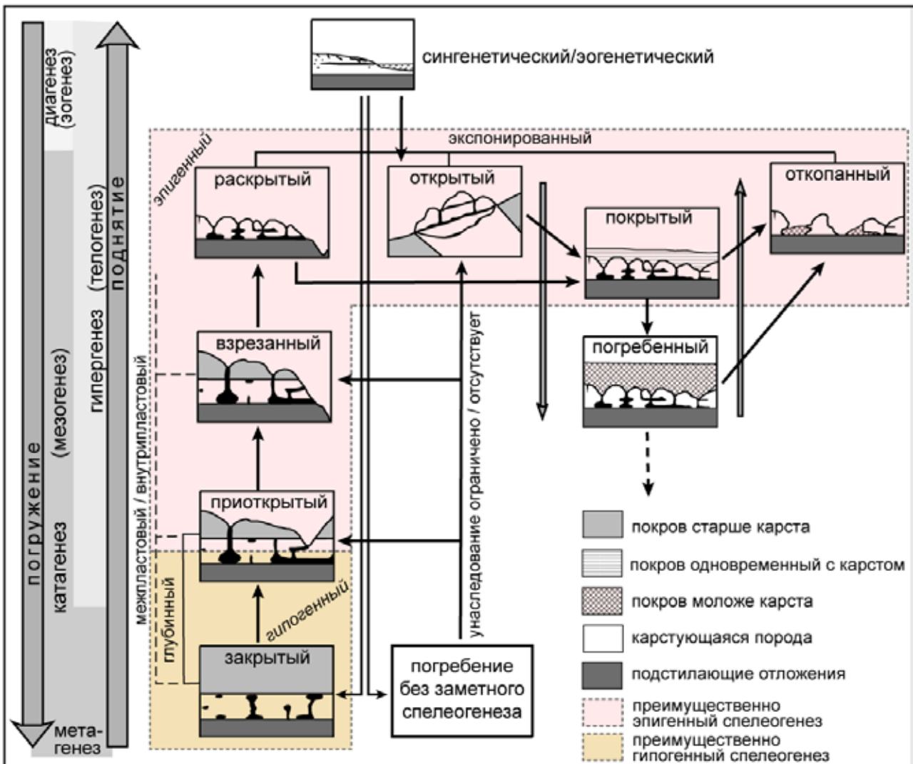
Рис. 2. Эволюционная классификация типов карста (по Klimchouk, 1996, с дополнениями).
