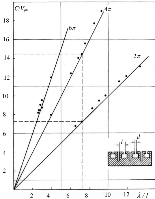
Рис. 1. Линии равных фазовых сдвигов \varphi = n\pi в координатах (C/V_{ph}; \lambda/l) и фрагмент продольного сечения периодической структуры. Точками нанесены результаты эксперимента
