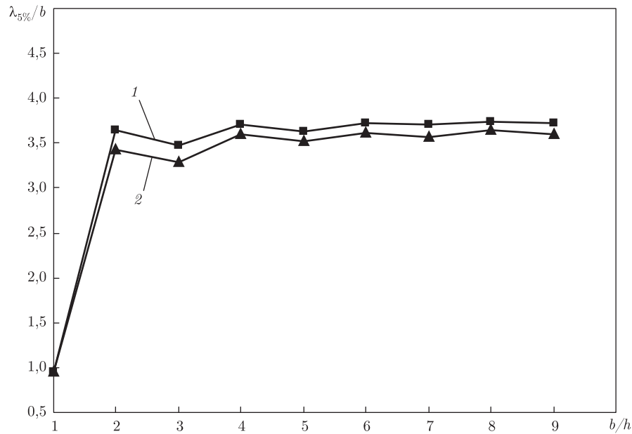
Рис. 2. Зависимость максимальной относительной протяженности \lambda_{5\%}/b зоны краевого эффекта от периода поверхностной нагрузки b : 1 — материал без покрытия; 2 — материал с покрытием
