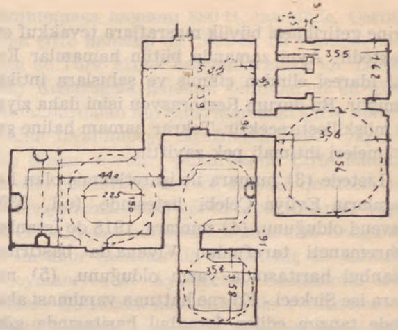
Istanbul — Hoca paşa hamamı kadınlar kısmının plânı Plan de la partie réservée aux femmes des bains de Hodjapacha
