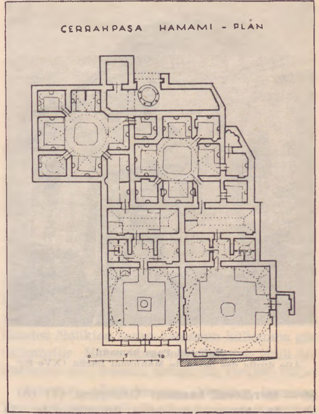
İstanbul — Cerrahpaşa hamamının plânı Istanbul — Plan des bains turcs de Djerrah Pacha
