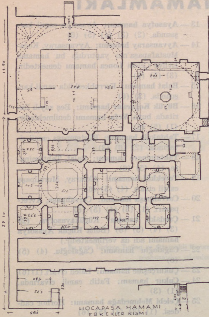
Istanbul — Hoca Paşa hamamı erkekler kısmının plânı Plan de la partie réservée aux hommes des bains de Hodjapacha
