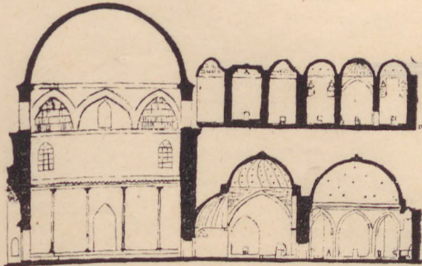
Mahmud Paşa hamamının kesiti Coupe des bains de Mahmoud Pacha
