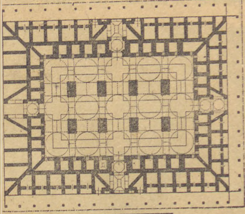
Bedestenin plânı
