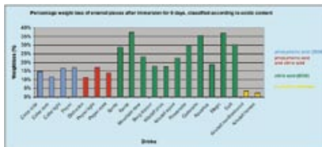
Tafla 2. Meðal þyngdartap tannhluta í mismunandi gosdrykkjasýnum flokkaðir í fjóra meginhópa eftir sýrutegund þeirra. Table 2: Average weight loss of tooth pieces in the different drinks classified into four groups according their acid content.
