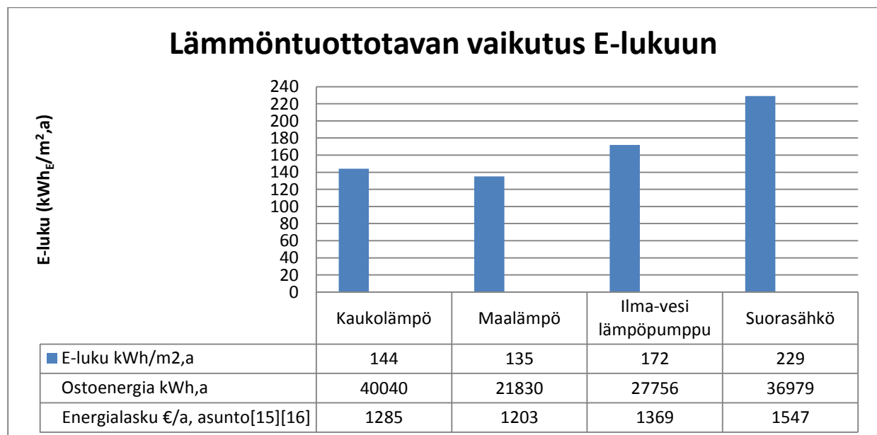
Kuva 8. Lämmöntuottotavan vaikutus rakennuksen E-lukuun
