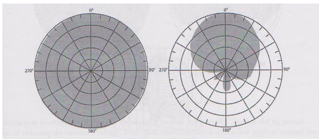
KUVA 10. Antennien luomat kuviot horisontaalisesti kuvattuna, vasemmalla on ympärisäteilevän antennin kuvio ja oikealla suunnatun antennin kuvio (Salter 2013, 35.)
