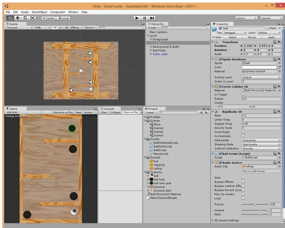
Kuva 1. Editorin päänäkymä
