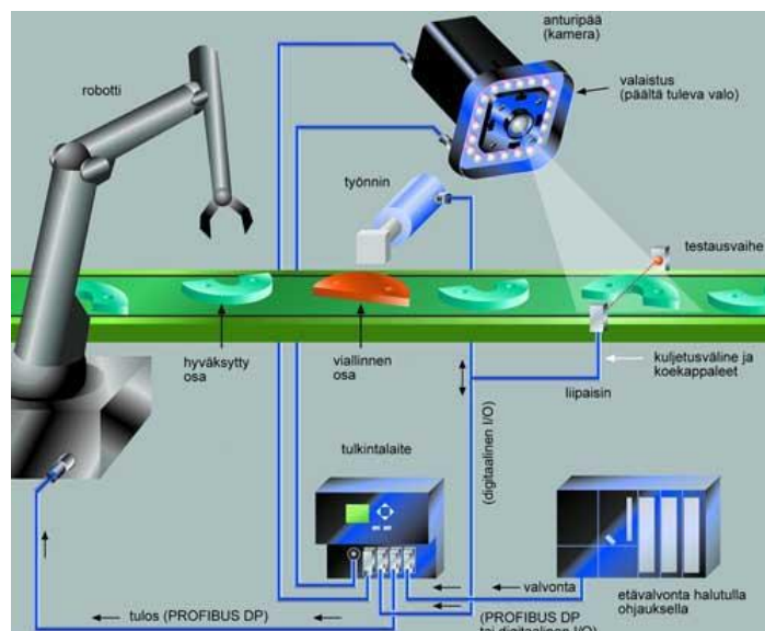
Kuva 3. Kamerajärjestelmän koostumus. /2/
