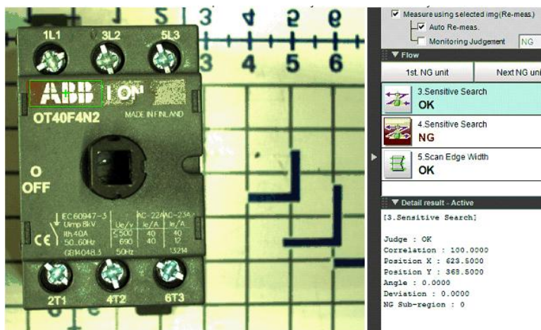
Kuva 15. Sensitive search. /11/
