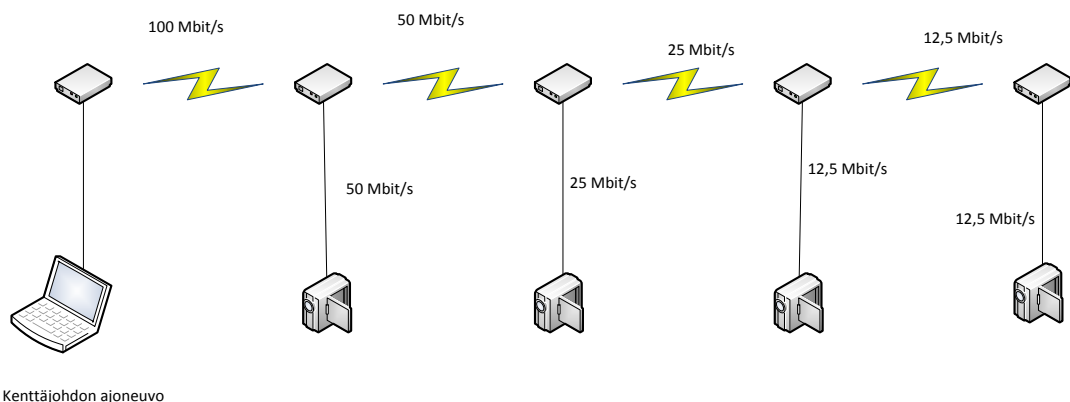
Kuva 15. Tiedonsiirtokaistan puolittuminen.
