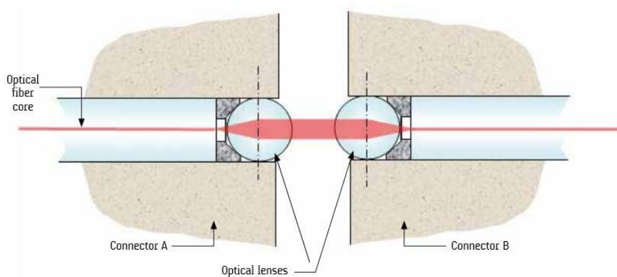
Kuva 6. Valoa kuljetavan ytimen pinta-alan kasvattaminen linssien avulla [11].
