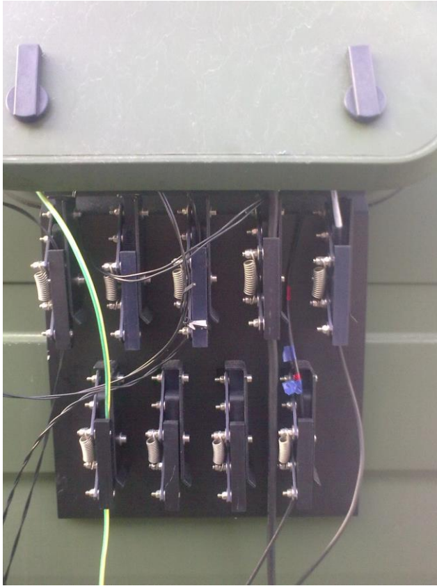
Kuva 24. Vedonpoistopaneeli.
