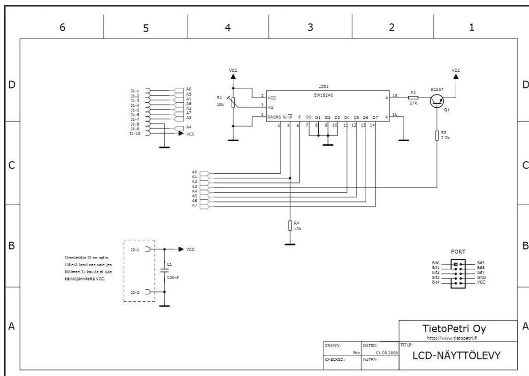
Kuva 5. LCD-näyttölevyn kytkentäkaavio. (LCD-näyttölevyn kytkentäkaavio, 1.4.2013)
