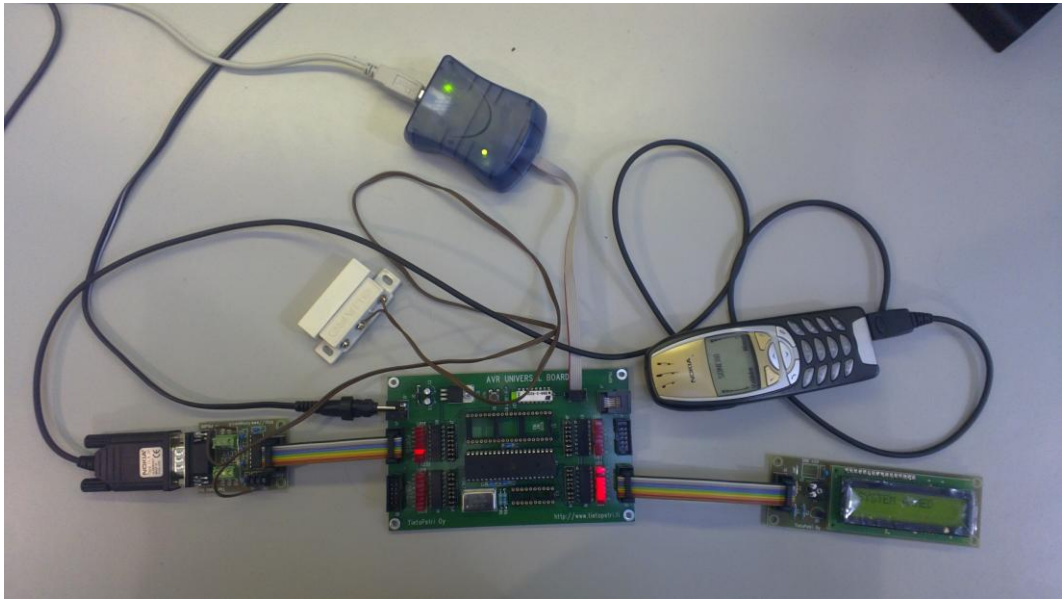
Kuva 18. Murtohälytin.
