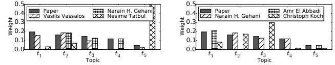
(c) Greedy (Score = 0.87) (d) SDGA-SRA (Score = 0.96)
