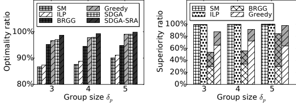
(c) Optimality ratio (DB) (d) Superiority ratio (DB)
