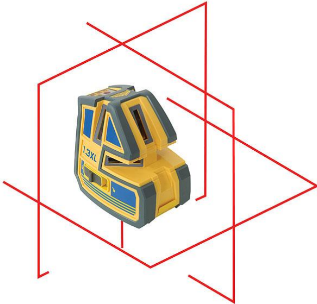
Kuva 14. Ristiviivalaser (Geotrim4 2012)
