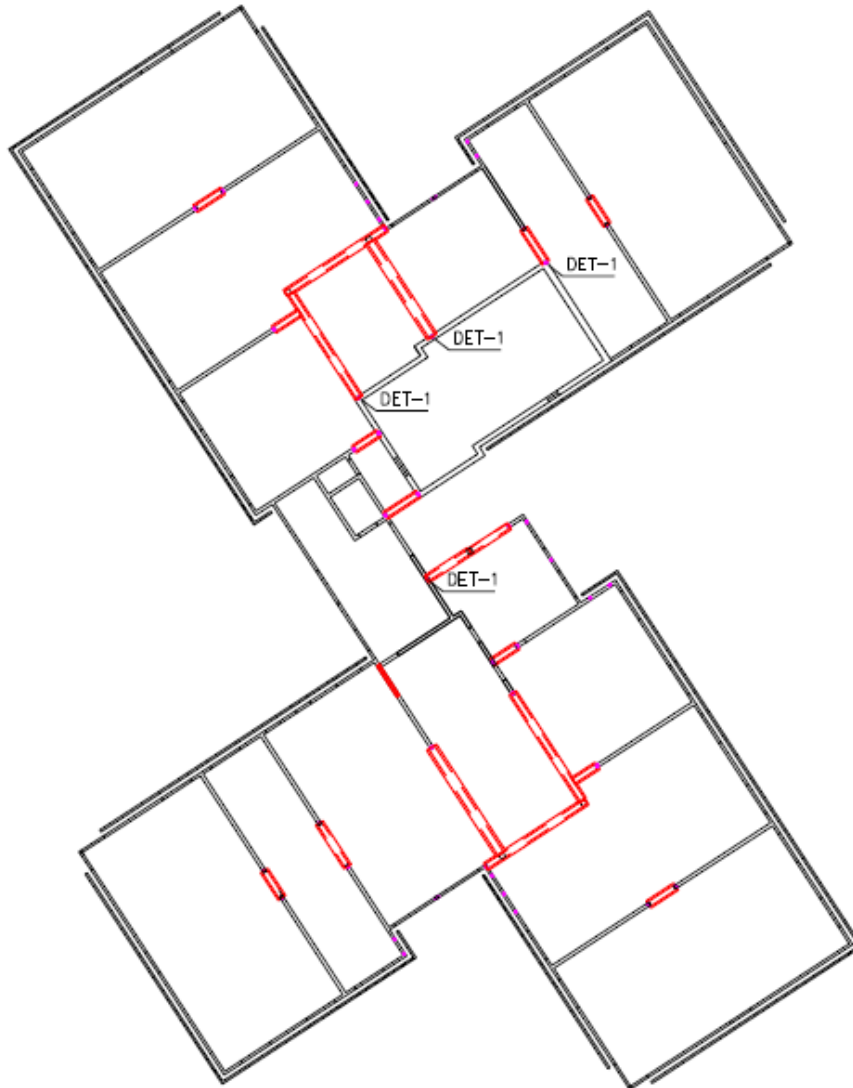
Kuva 22. Deltapalkkien paikat rautalankamallina.
