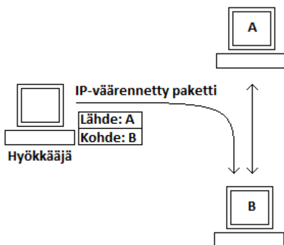
KUVA 7. IP-väärennöksen toiminta
