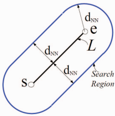
Fig. 12. |PNN(\mathcal{L})|
