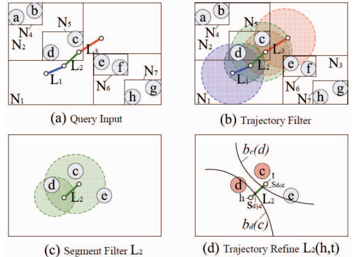
Fig. 7. TPNNQ
