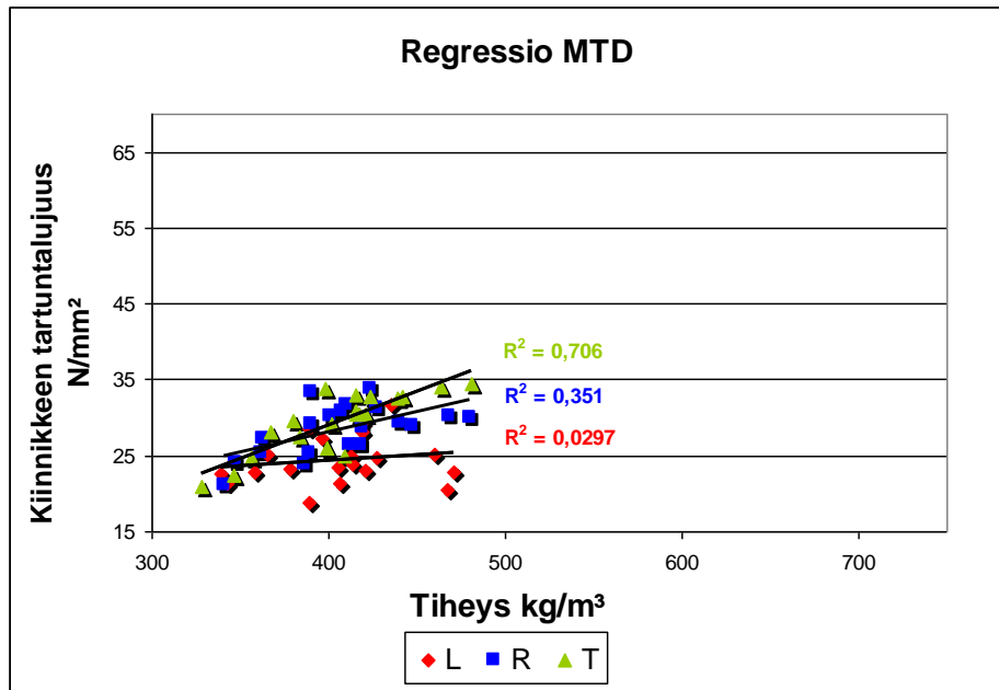
Kuva 12 Regressio MTD.
