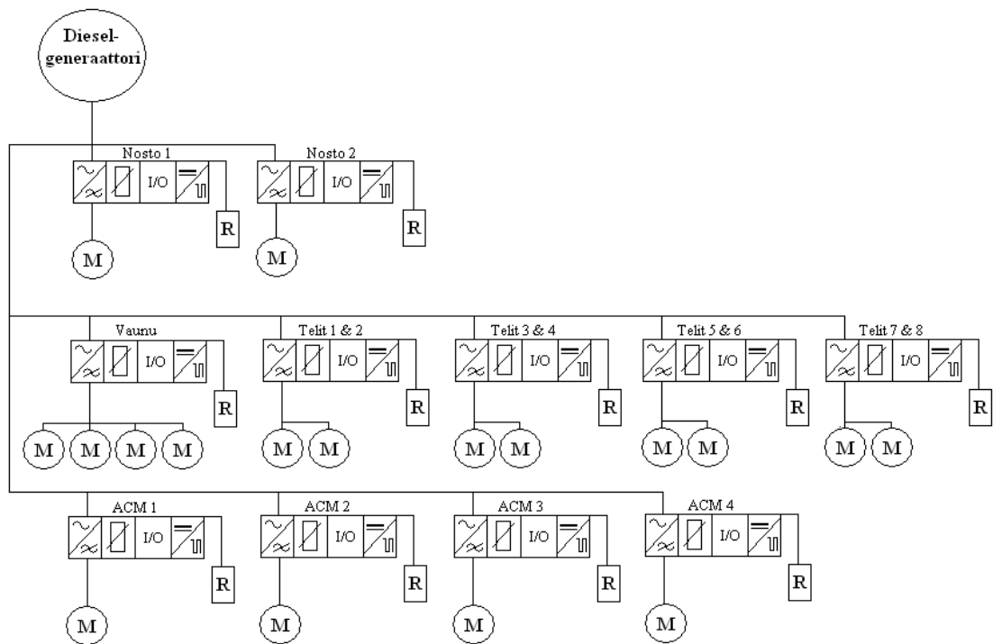
KUVA 15. Periaatekuva modernisoidun RTG-nosturin taajuusmuuttajien kytkennästä.
