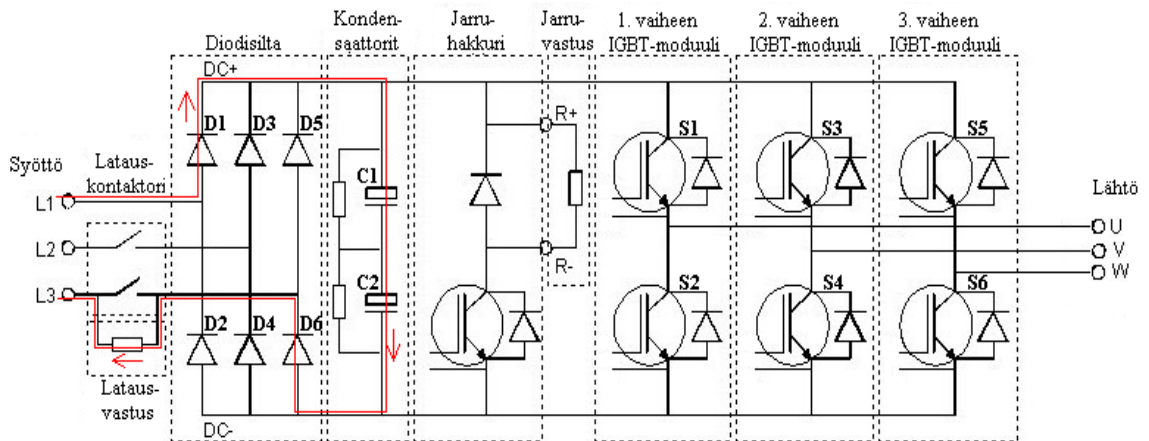
KUVA 5. DAV-taajuusmuuttajan kaaviokuva. [12]
