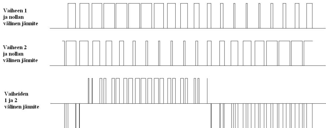
KUVA 7. Pulssinleveysmodulaation periaate. [5. s.131.]
