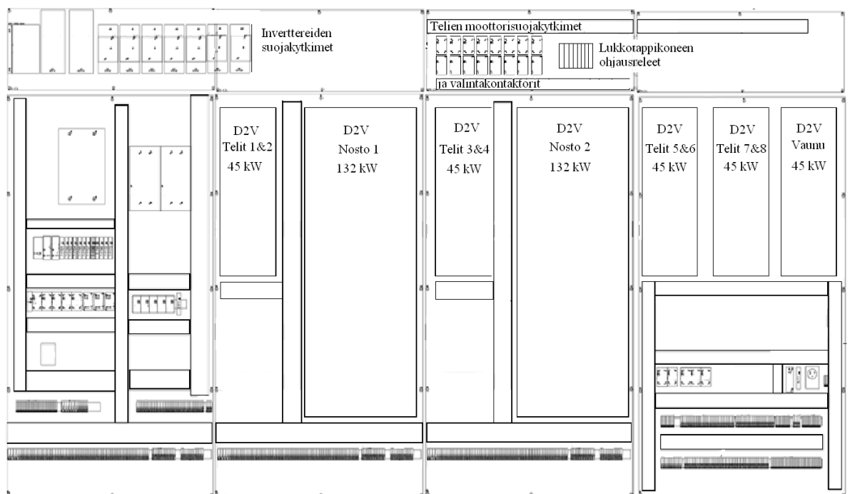
KUVA 17. Sähköhuoneen komponenttien sijoittelu.
