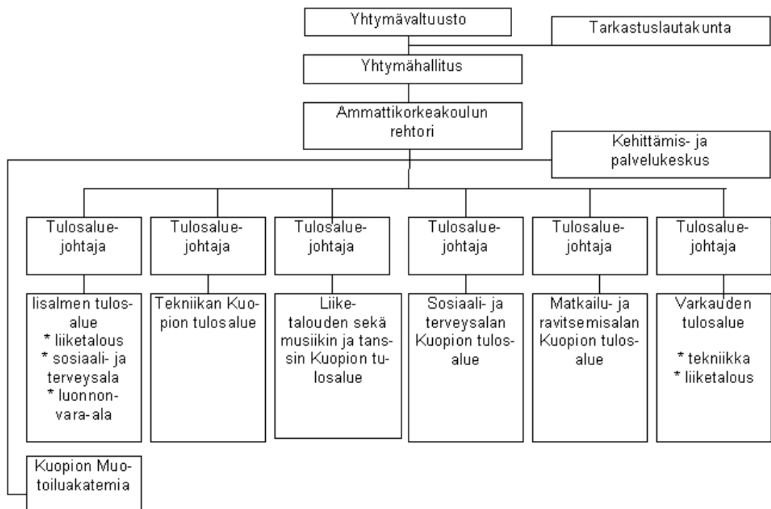
Kuva 1. Savonia-AMK:n organisaatiokaavio.
