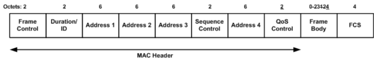
Kuva 1 802.11 MAC-kehys (3, s. 60.)
