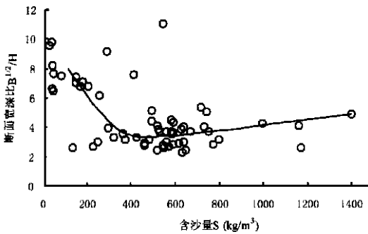
图 3 流量大于 500 \text{ m}^3/\text{s} 时含沙量(S)与断面形态( B^{1/2}/H )关系
