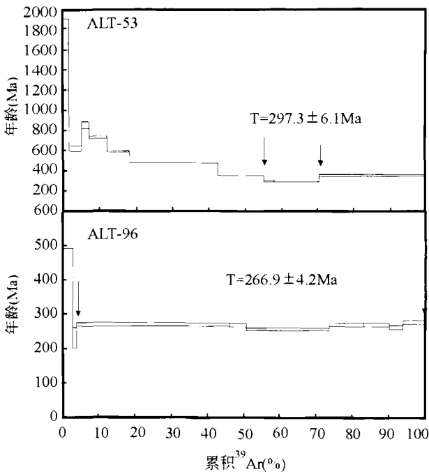
图 2 斜长角闪岩和辉长岩的 40 Ar- 39 Ar 表现年龄
