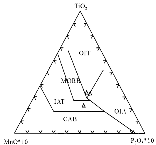
图8 塔尔浪斜长角闪岩 TiO 2 -MnO-P 2 O 5 判别图 (Pearce and Cann, 1973) (图中: CAB-大陆弧玄武岩; MORB-洋中脊玄武岩; IAT-岛弧拉斑玄武岩; OIT-洋岛拉斑玄武岩; OIA-洋岛碱性玄武岩)
