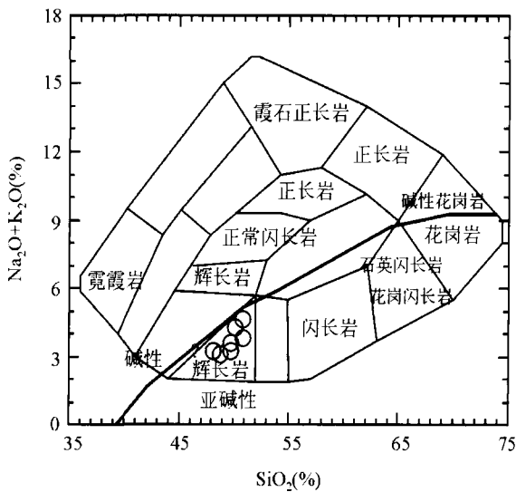
图6 塔里木辉长岩 (Na 2 O + K 2 O)-SiO 2 图解 (Cox, 1979)
