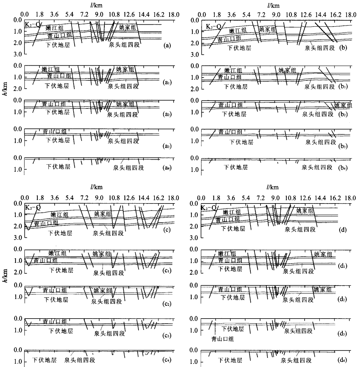
图 2 剖面 1- 4 的平衡地质剖面 (a, b, c, d) 及反演构造剖面 (a 1 - d 4 )
