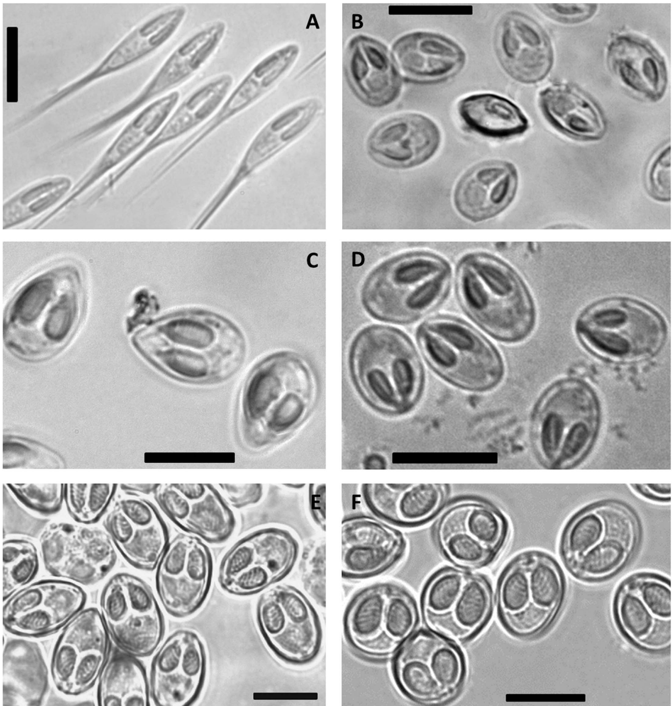
Figure 1. Photomicrographs of fresh spores of the novel myxosporean species. (A) Henneguya maculosus n. sp.; (B) Myxobolus flavus n. sp.; (C) Myxobolus aureus n. sp.; (D) Myxobolus pantanalis n. sp.; (E) Myxobolus umidus n. sp.; (F) Myxobolus piraputangae n. sp. Scale bars = 10 \mu m. doi:10.1371/journal.pone.0073713.g001
