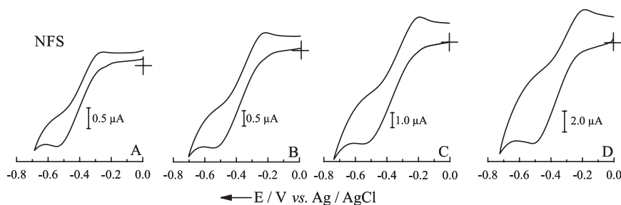
Figure 5. Cyclic voltammograms recorded at pH 10.01. [NFS] = 0.5 mmol L -1 . (A) 0,02 V s -1 ; (B) 0,05 V s -1 ; (C) 0,1 V s -1 ; (D) 1,0 V s -1 .
