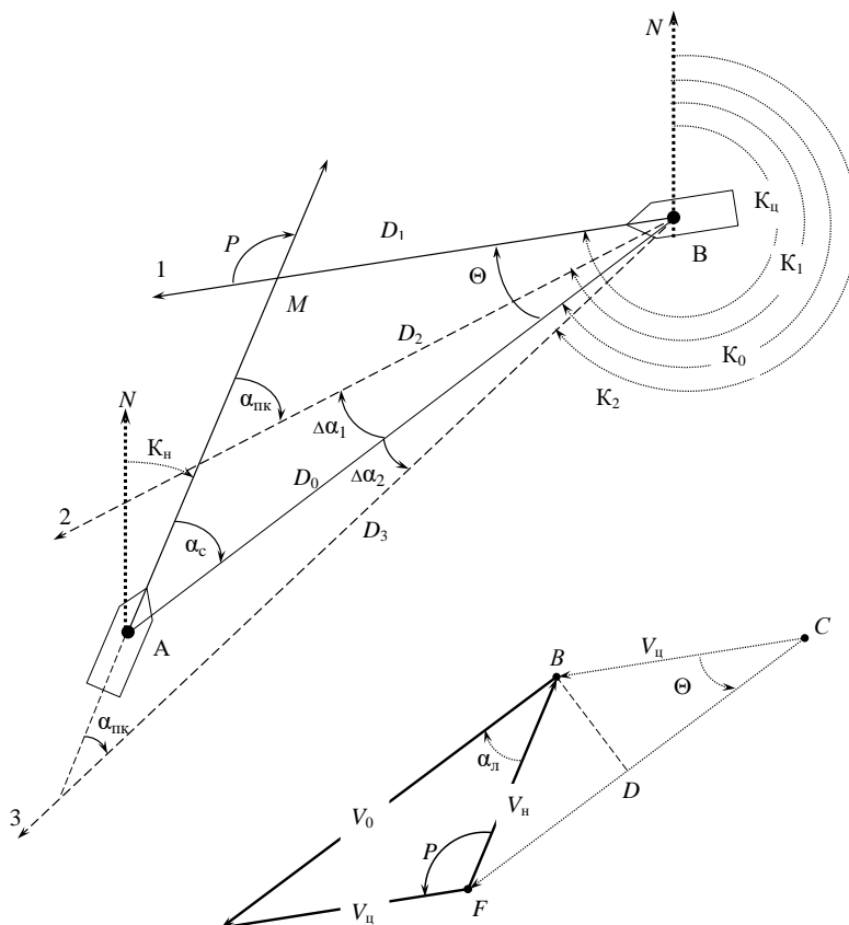
Рис. 1. Оцінка безпеки зіткнення за зміною кута курсу ліній відносного руху
