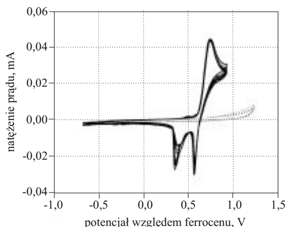
Rys. 2. Przebieg CV podczas elektrotleniania monomeru A (—) w dichlorometanie w obecności soli elektrolitu Bu_4NBF_4 (●●●●)
