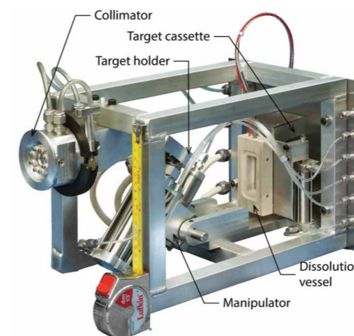
Fig. 2- Sistema integrado para a irradiação e dissolução de alvos sólidos. http://www.advancesystems.ca/
