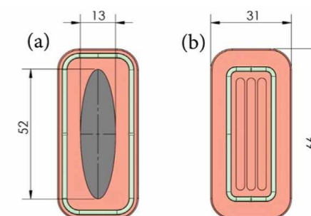
Fig. 3- Alvo sólido, frente e verso; (a) mostra a área irradiada frontal a cinzento e o substrato a laranja; (b) mostra os canais de arrefecimento. As dimensões estão em mm.
