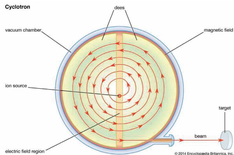
Fig. 1- Principais componentes e modo de funcionamento de um ciclotrão.
