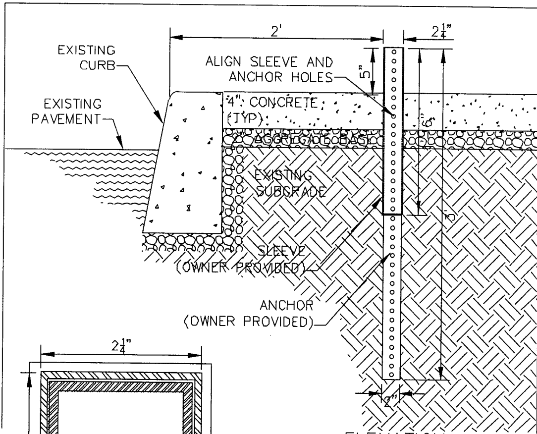
ELEVATION SCALE: 1/2" = 1"
