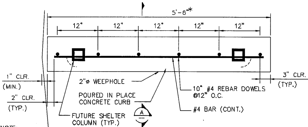
PLAN DETAIL SCALE: 1" = 1'-0"
